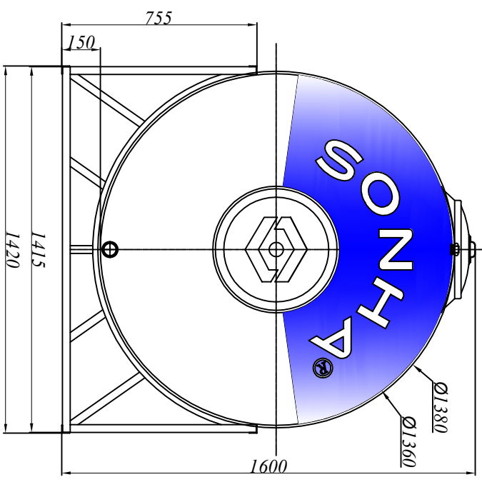
HÌNH CHIẾU A-A
