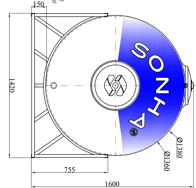
MẶT CHIẾU A-A
