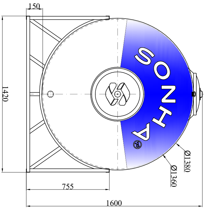
MẶT CHIẾU A-A
